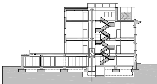
longitudinal section A-A'
